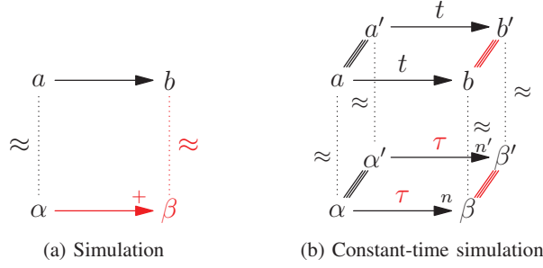
Fig. 5: Manysteps simulations
