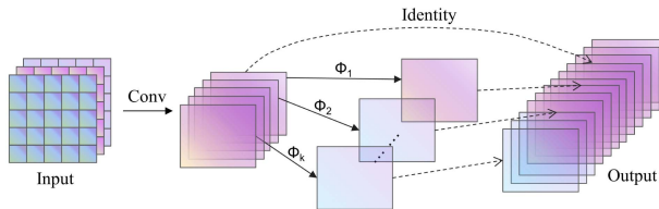
(b) The Ghost module.
